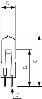
6550 150W G6.35 15V
